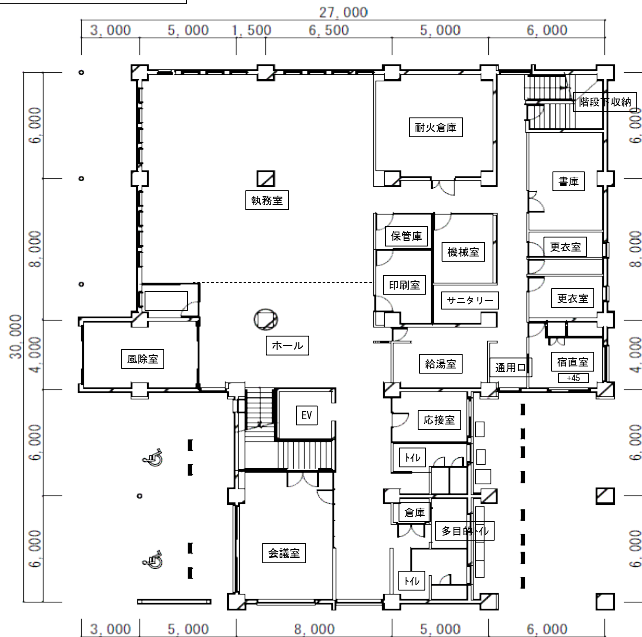
1階平面図（新小代地域局）
