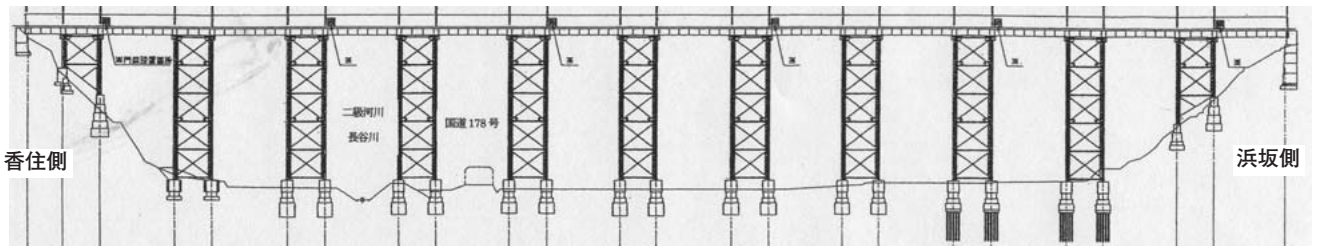
余部鉄橋 橋梁一般図（側面図）
