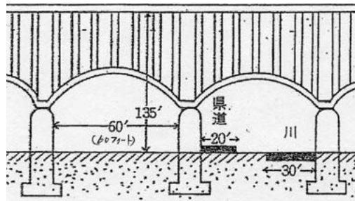
当時の鉄筋橋案
