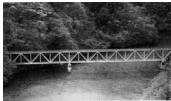
▲第三只見川橋梁〔JR只見線〕 上路ワーレントラス橋、長さ180m 昭和31年(1956)完成
