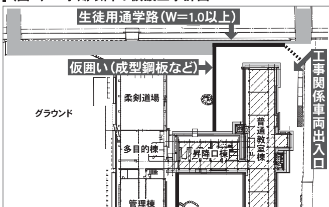
【図2】2学期以降の仮設工事計画
