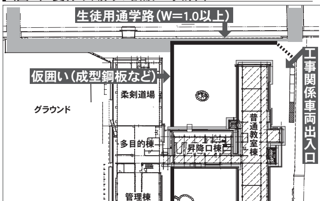
【図1】夏休み期間の仮設工事計画
