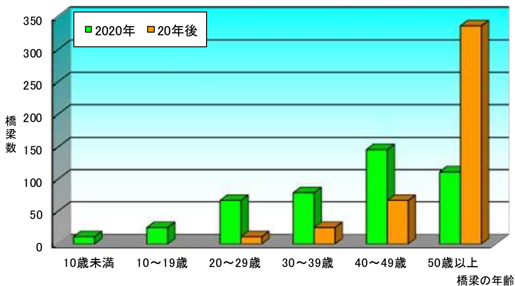
高齢化橋梁の割合の変化
